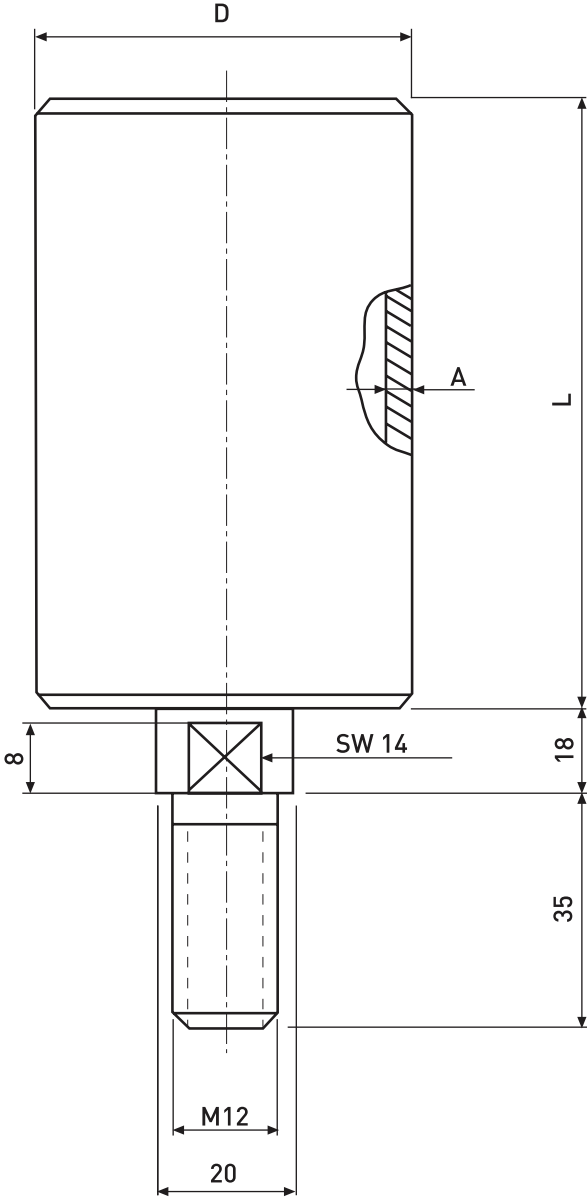
Guide roller
