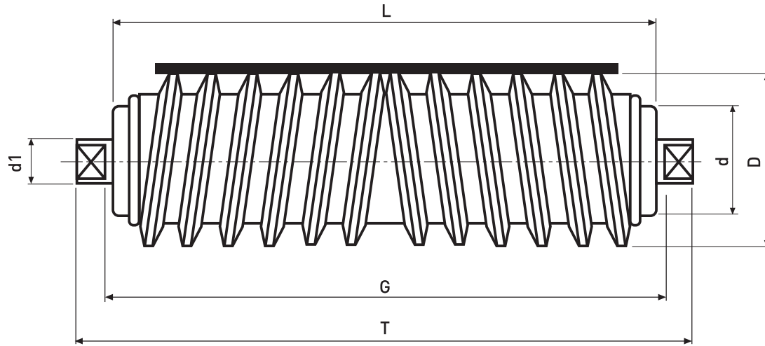
Helicoidal return roller.
